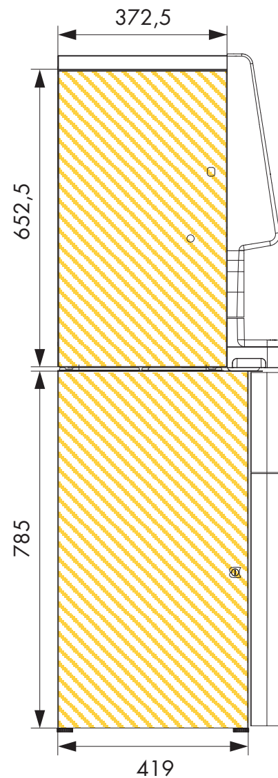
fianco sinistro left side
